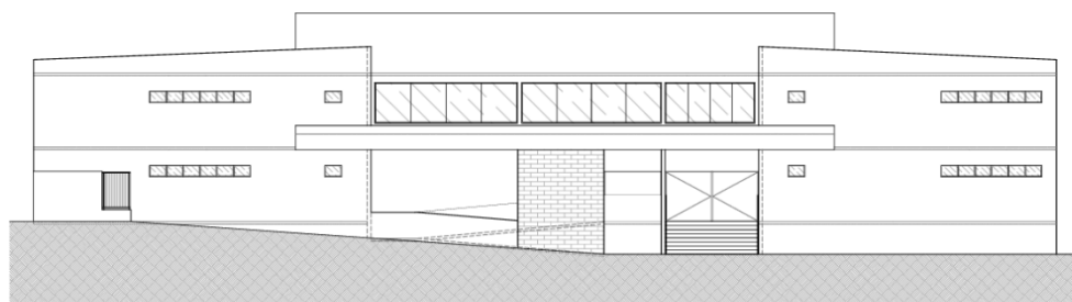
FACHADA FRONTAL ESCALA 1:150
