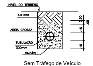
Detalhe Proteção de Tubulação Enterrada SEM ESCALA
