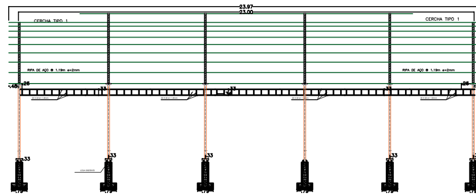
CORTE B-B DADOS Y ESTRUCTURA DEL TECHO ESC: 1/50
