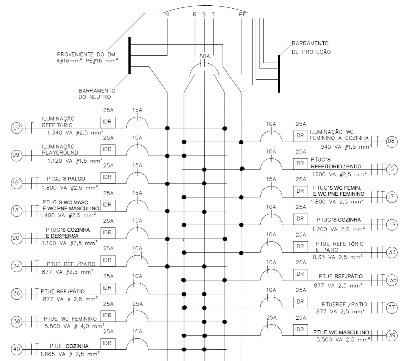
2 DIAGRAMA UNIFILAR CD II ESC.1/50
