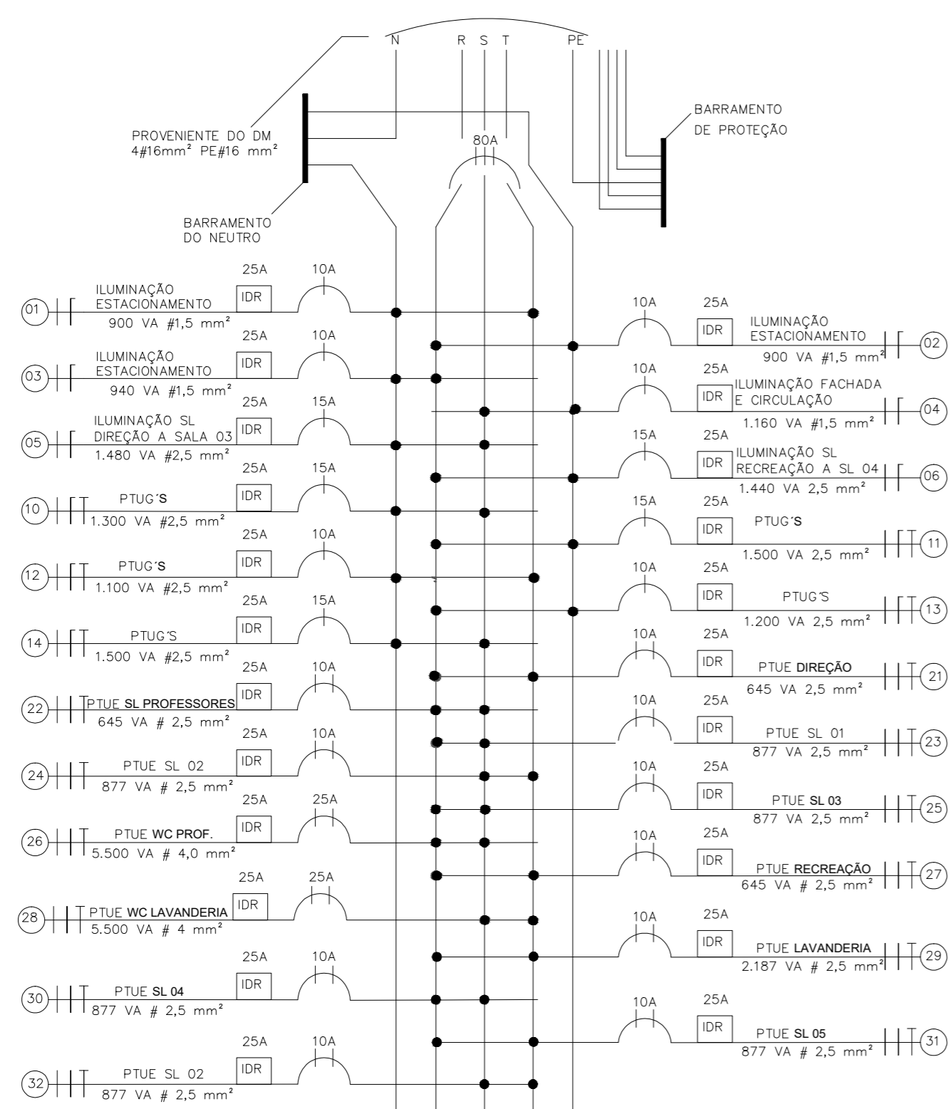
2 DIAGRAMA UNIFILAR CD I ESC.1/50
